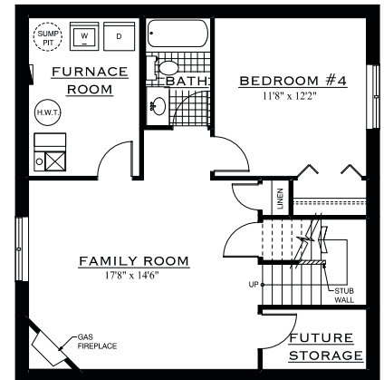
OPTIONAL BASEMENT PLAN 545 SQ.FT.
